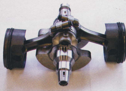
V-Motor mit kompakter Kurbelwelle und 75 Grad Zylinderwinkel. Den wassergekühlten Vierventiler zeichnet ein rennsportliches Layout aus. Nockentrieb ähnlich wie beim Suzuki-Twin über eine Kombination aus Kette und Stirnrädern
